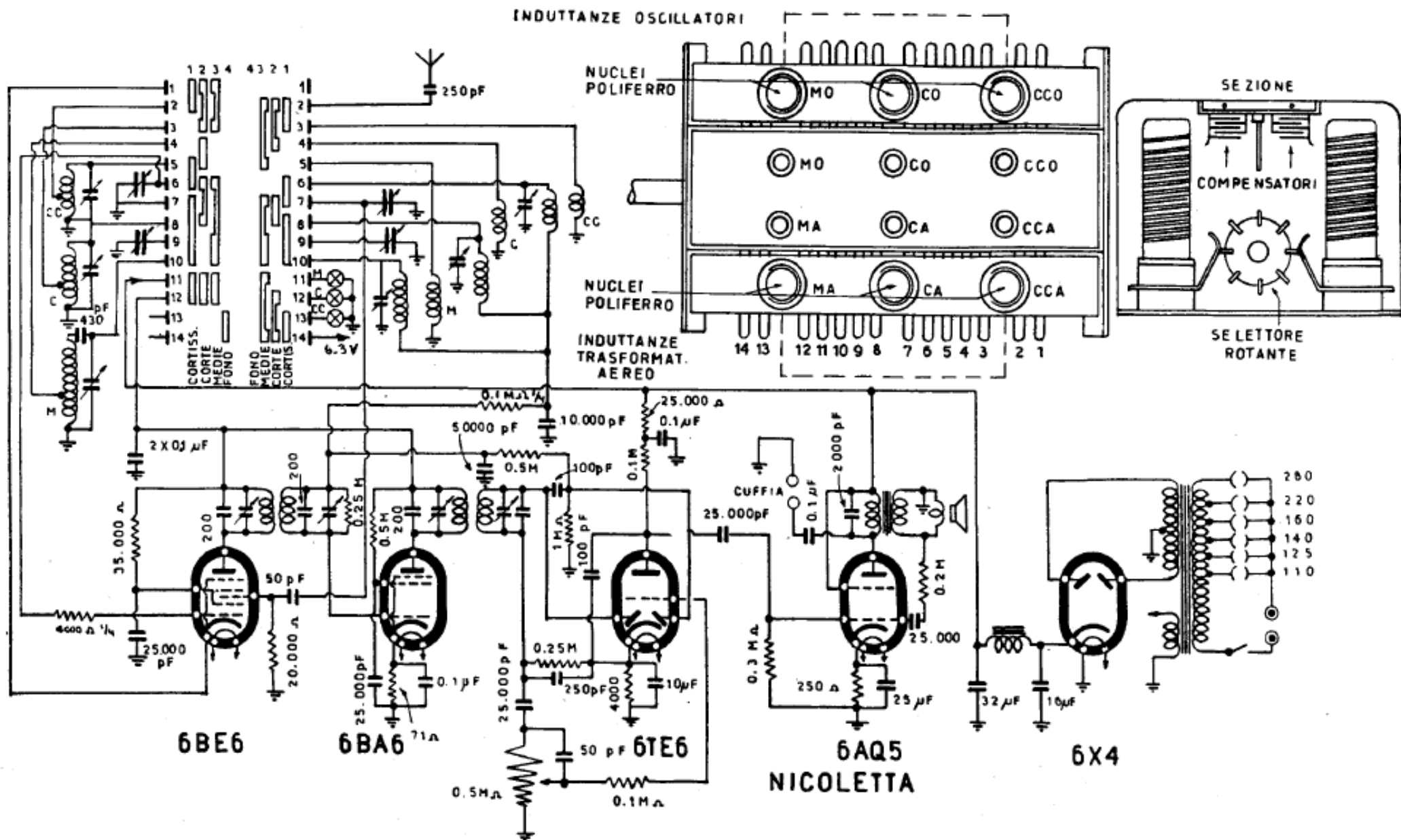
IMCARADIO - Mod. IF 51 « NICOLETTA » - Gamma onde medie intera, gamma onde corte-cortissime da 13 a 51 metri, con allargamento di banda continuo, mediante condensatore variabile e comando sintonia separati. Media frequenza 460 kc. Altoparlante a magneti permanente. Potenza d'uscita 4 watt.
